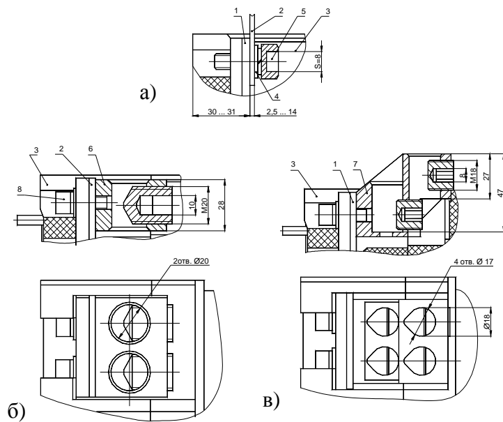
Рисунок 3 - Способы присоединения внешних проводников главной цепи выключателя.
