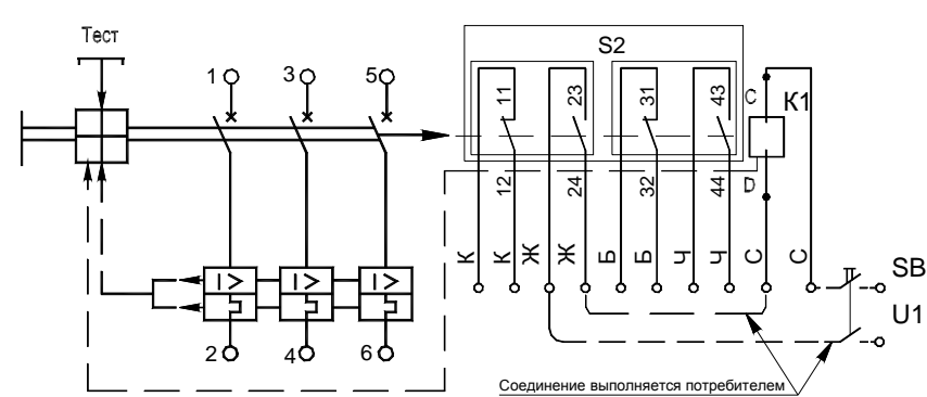
г) Выключатель с независимым расцепителем и вспомогательными контактами.
