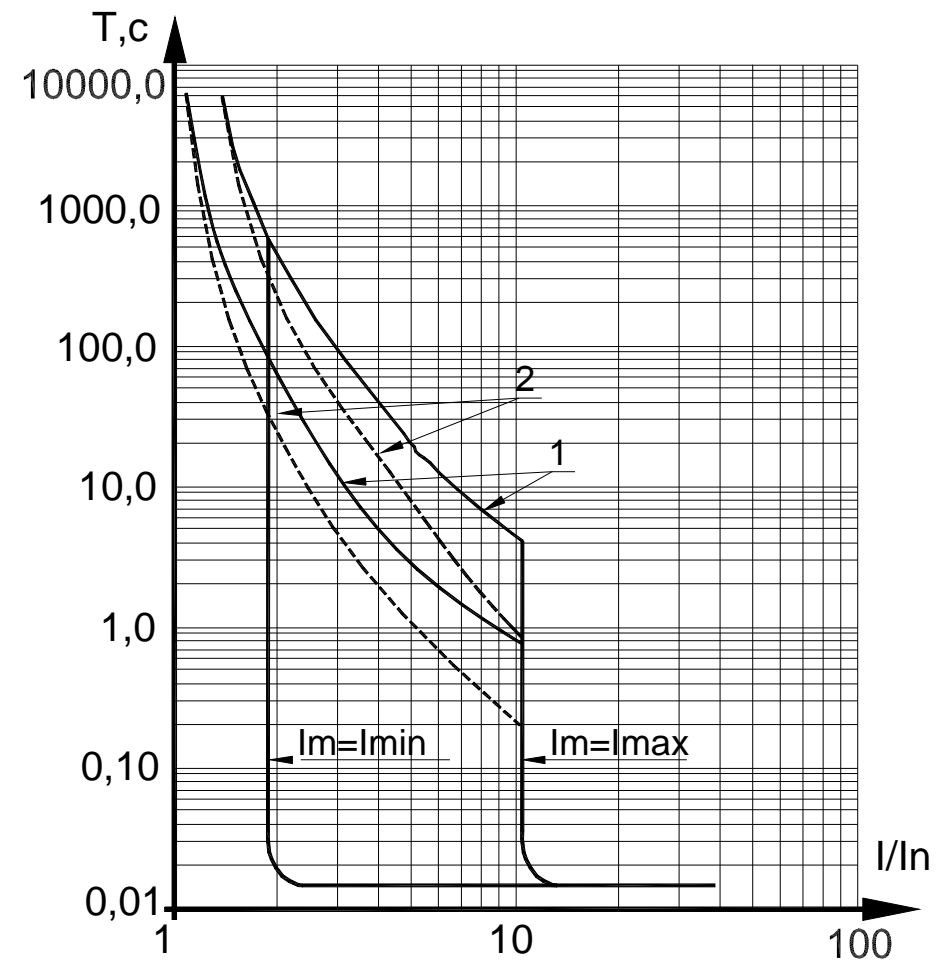
1 - зона работы теплового максимального расцепителя тока с холодного состояния 2- зона работы теплового максимального расцепителя тока с нагретого состояния
